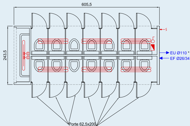
PLAN DU MODULAIRE 14 WC
