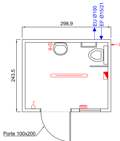
PLAN DU MODULAIRE PMR 1 WC (option douche)
